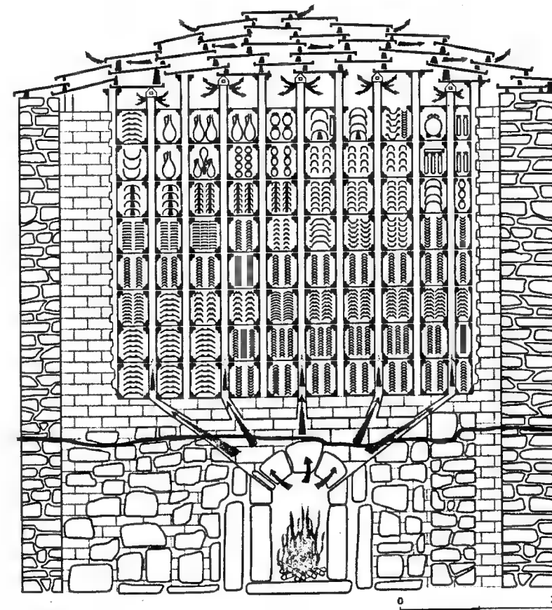
Kaiserzeitlicher Töpferofen von La Graufesenque (Aveyron), 1.-2. Jh. (Rekonstruktion A. Vernhet). 2 ■ hoch erh. Unterbau aus 80 cm dicken Steinmauern, mit zentralem Feuerungskanal, oberer Teil ergänzt. Mitgefündene Tontuben, Tonplatten (45 ■ 62 cm), Brennstützen und Fehlbrandstapel belegen die Rekonstruktion der Einsetzordnung des Brenngutes.
